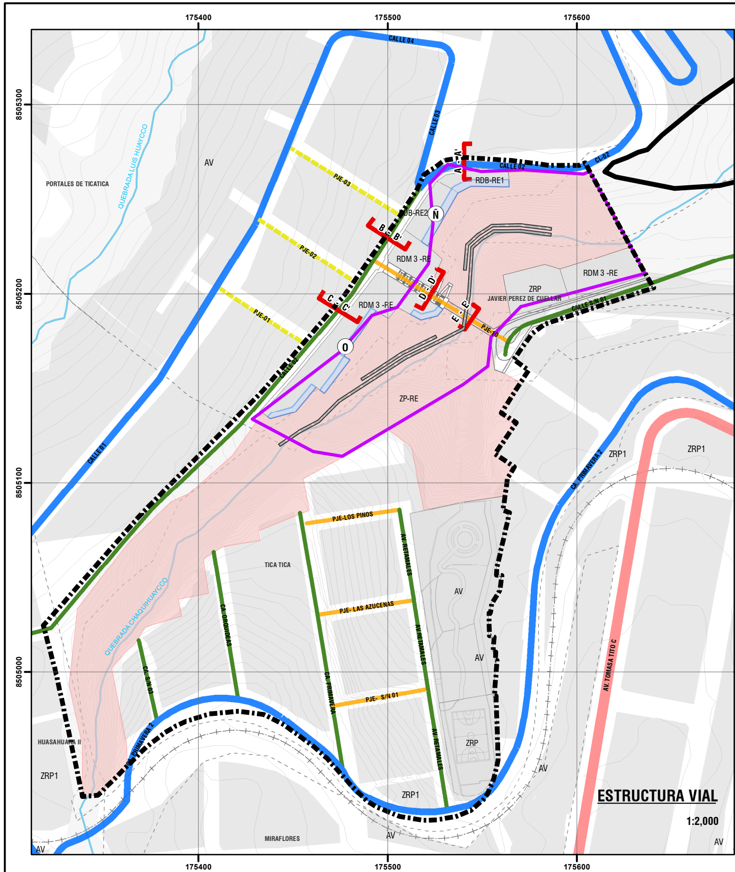
PUENTE PEATONAL - QUEBRADA "CHAQUIHUAYCCO"
